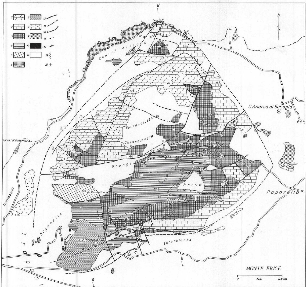
TAV. 1 —Carta geologica del Monte Erice.
