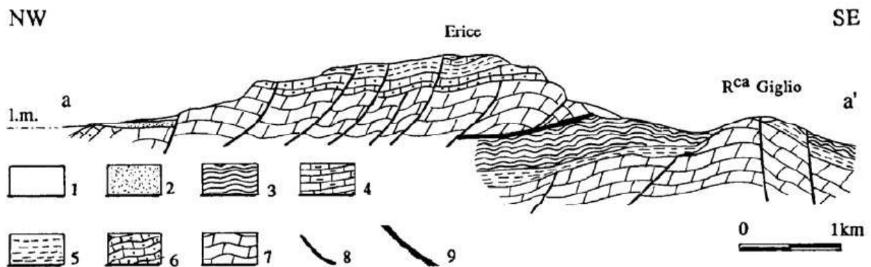
Legenda sezione geologica. 1) Detrito; 2) calcarenite, sabbia e conglomerati (Peistocene-Pliocene sup.); 3) calcareniti e biocalcareniti "Mischio"; argille, argille marnose, marne ed arenarie; calcilutiti e calcisiltiti marnose "Scaglia" (Tortoniano-Cretaceo sup.); 4) calcilutiti e calcisiltiti a calpionelle "Lattimusa"; calcareniti e calciruditi ad Orbitoline (Neocomiano-Titonico); 5) calcari nodulari ad ammoniti "Rosso Ammonitico" (Malm-Dogger sup.); 6) calcilutiti a liste e noduli di selce (Dogger-Lias sup.); 7) dolomie, calcari dolomitici e calcari stromatolitici e loferitici (Lias-Trias sup.); 8) faglie; 9) superficie di sovrascorrimento.
